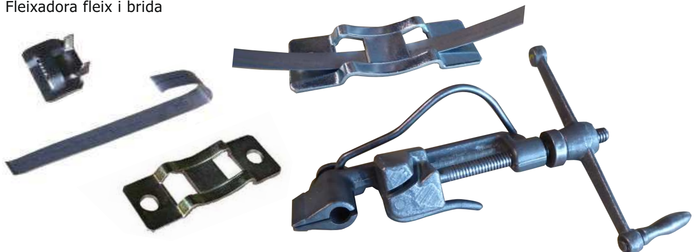
Fleixadora fleix i brida
